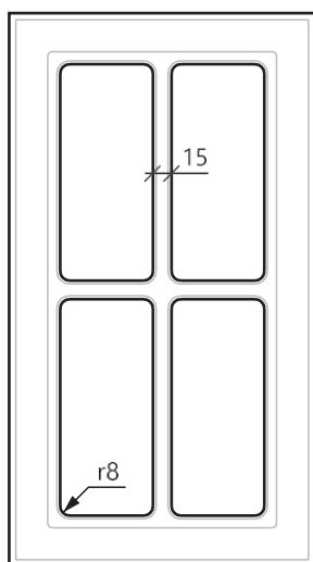
Минимальные размеры с фрезеровкой
